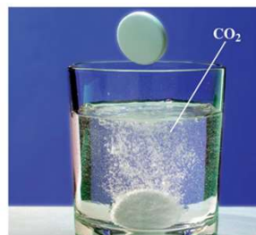
NaHCO 3
