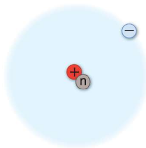
Deuterium 1 proton 1 neutron
